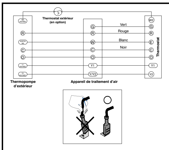
Figure 5. Raccordements de thermostat pour SH1BF4M2SX appareils de 5 tonnes
