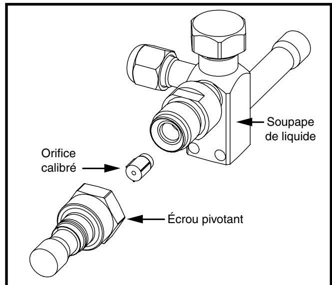
Figure 2. Soupape de liquide, orifice calibre et écrou pivotant
