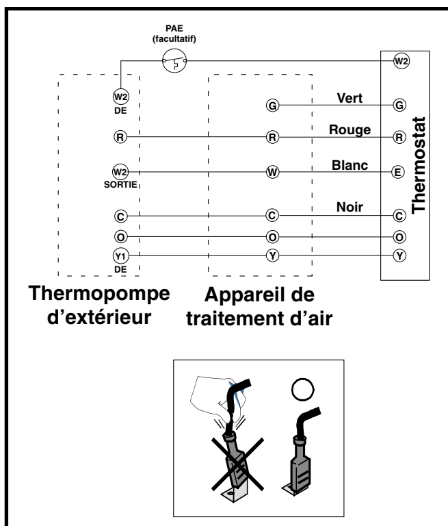
Figure 4. Raccordements de thermostat pour SH1BF4M1SP appareils de 2 - 4 tonnes
