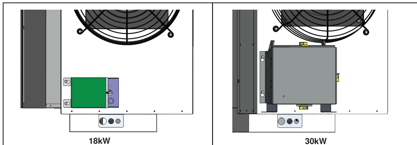
Figure 10. Installation d'un transformateur de 600V
