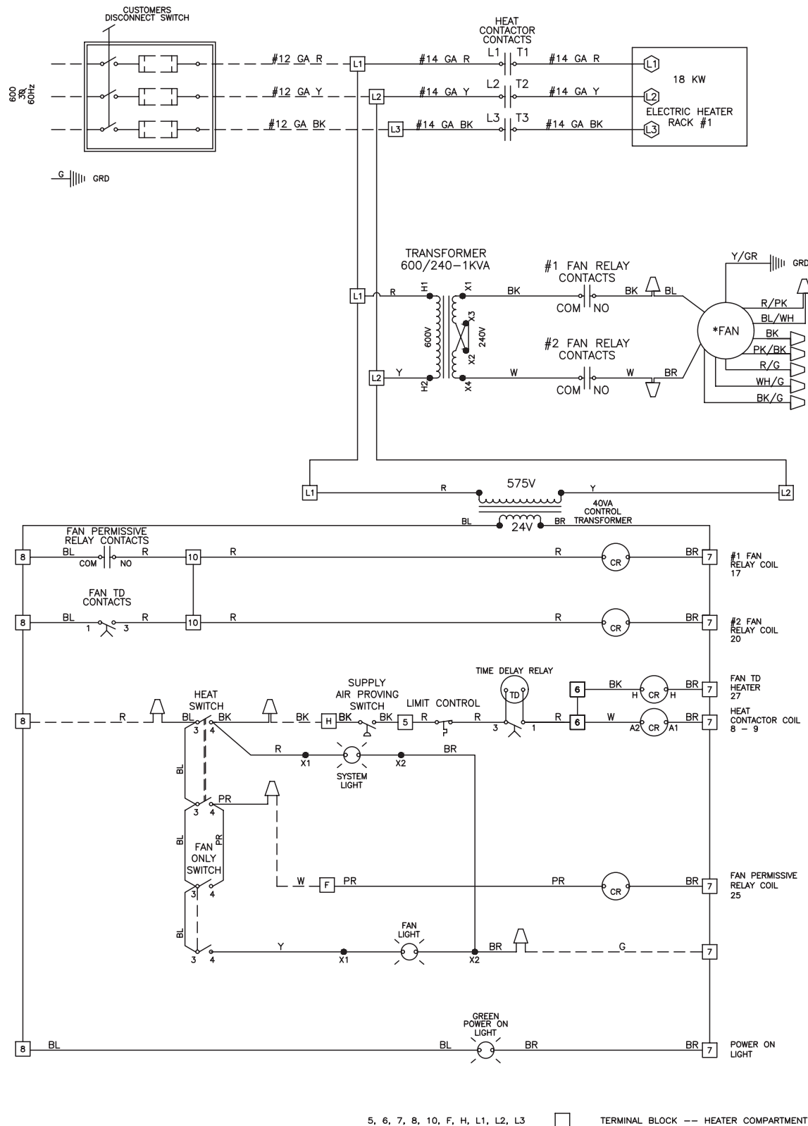
Schéma de câblage AK8E pour unité 600V 18kW
