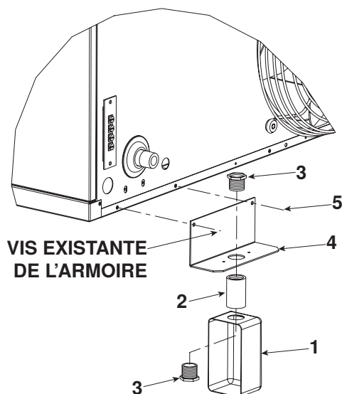
Figure 1. Kit de support de thermostat typique (se référer au Tableau 1)
